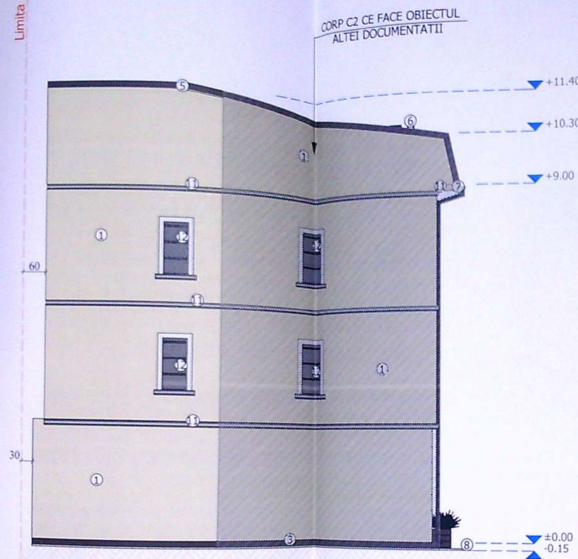
FATADA VEST PROPOS scara 1:100
