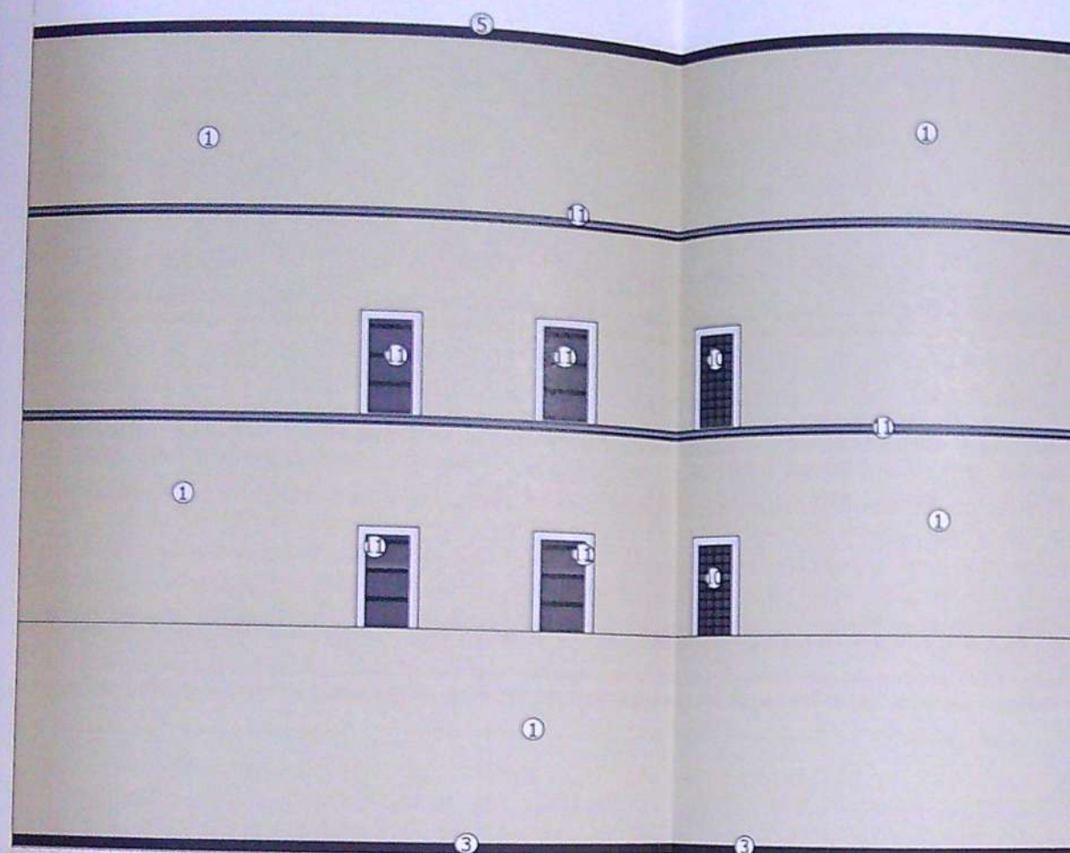
FATADA NORD PROPOS scara 1:100
